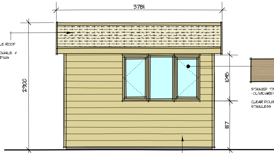
ELEVATION - B
