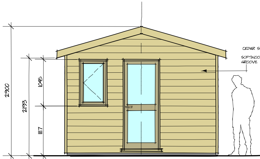
ELEVATION - A
