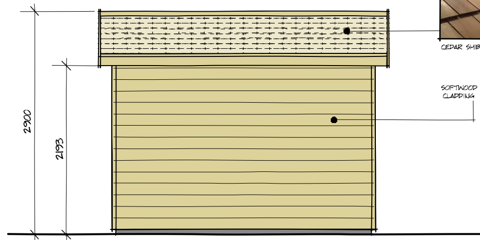
ELEVATION - D
