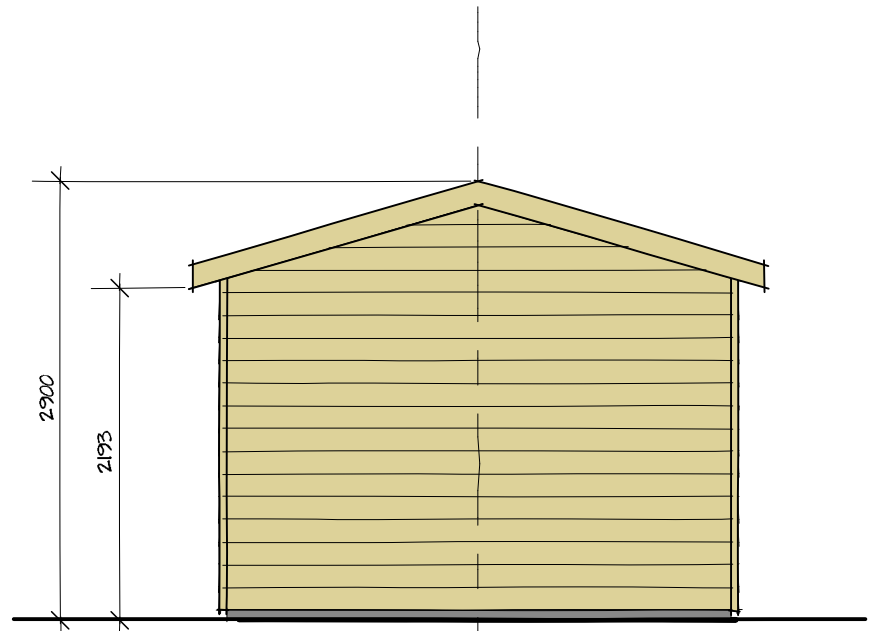
ELEVATION - A
