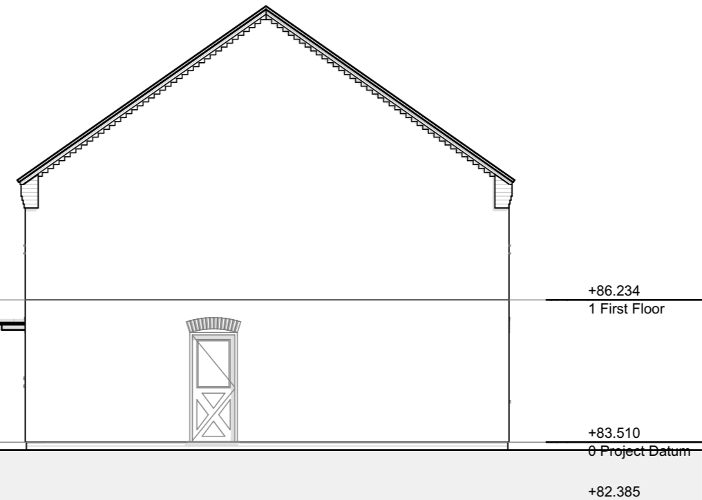
01-02 RIGHT ELEVATION 1:100
