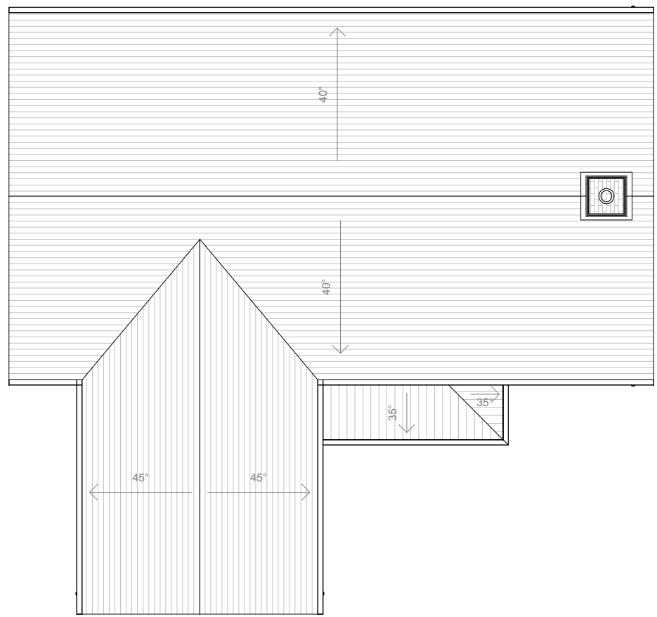
ellesworth cottage roof plan 1 : 100
